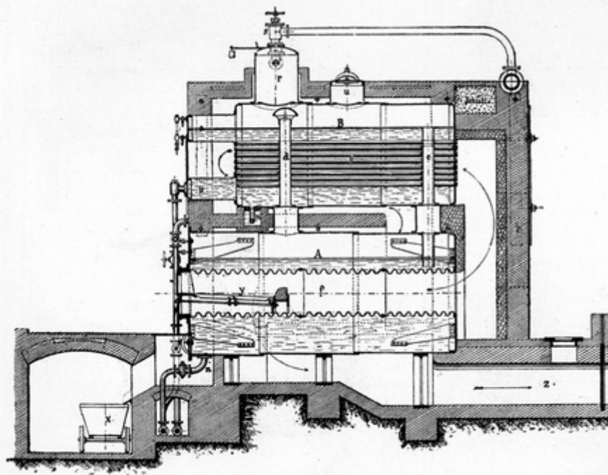
Fig. 119.—Longitudinal Section.
