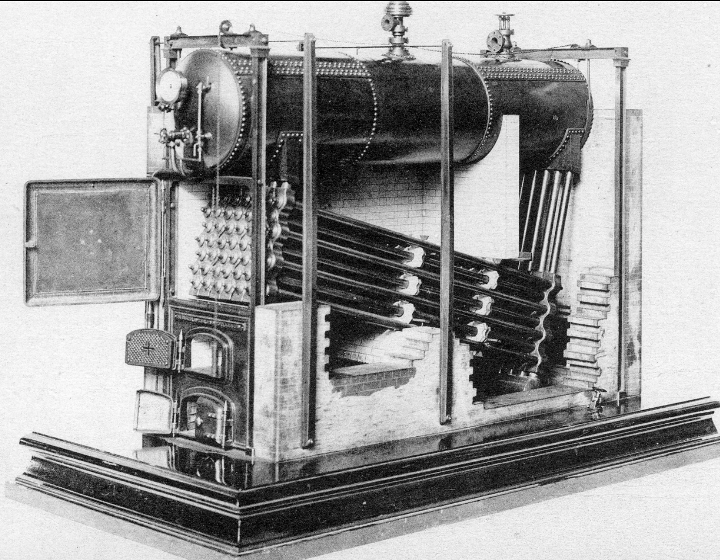
N° 11687. — Chaudière à vapeur à tubes d'eau système Babcock et Wilcox B-49
